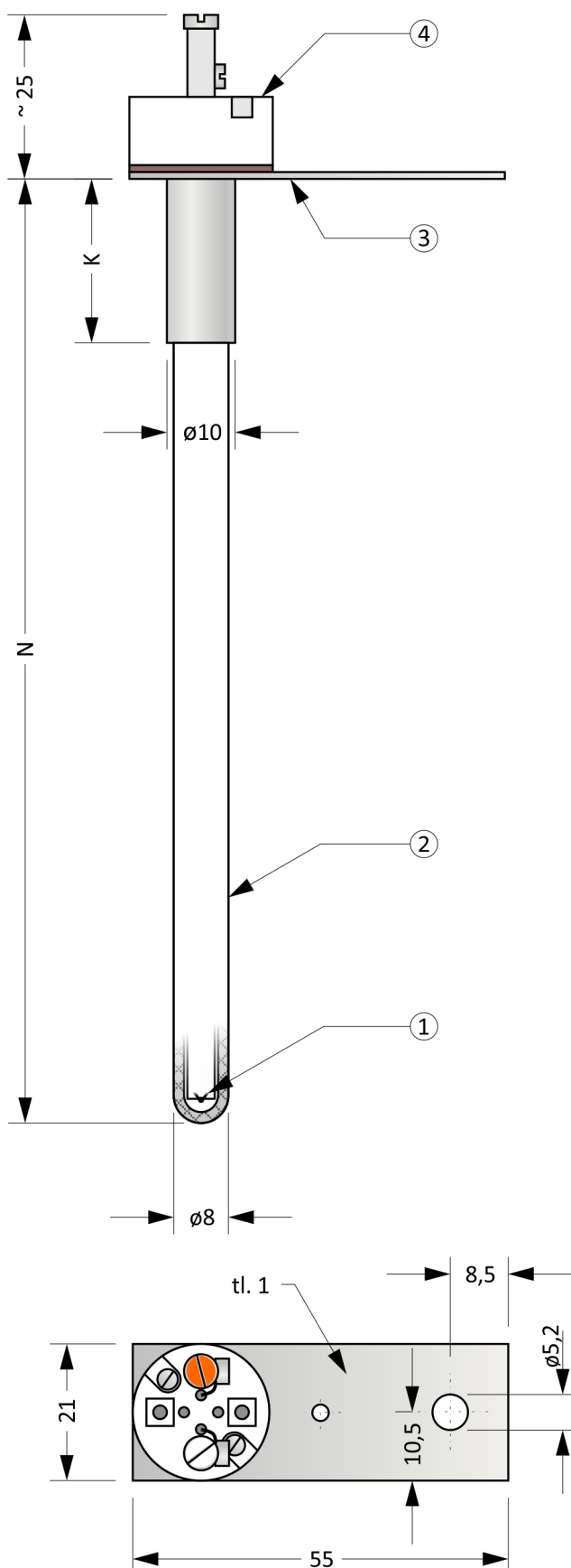
Obrázek 20.1: Snímač MTC20
