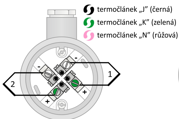
Obrázek 7.3: zapojení dvojitého termočlátku
