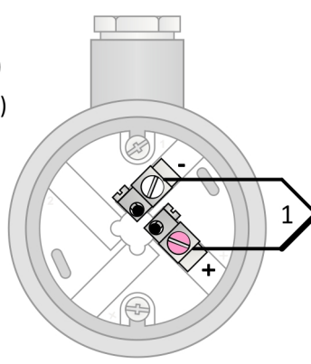
Obrázek 7.4: zapojení jednoduchého termočlátku
