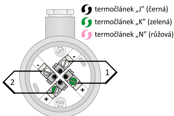
Obrázek 3L.3: zapojení dvojitého termočláнку
