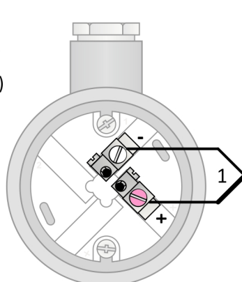
Obrázek 3L.4: zapojení jednoduchého termočláнку
