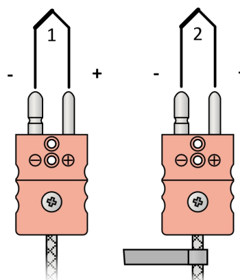
Obrázek 1KD.6: zapojení dvojitého termočláneku se dvěma konektory
