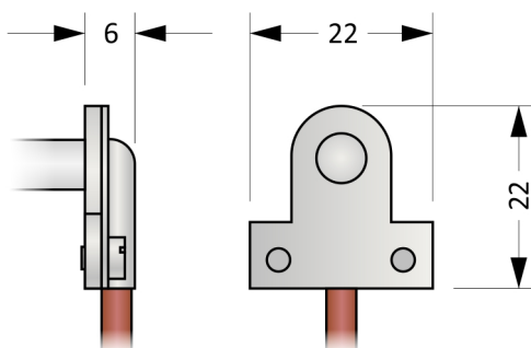
Obrázek 12U.2: Detail přechodky
