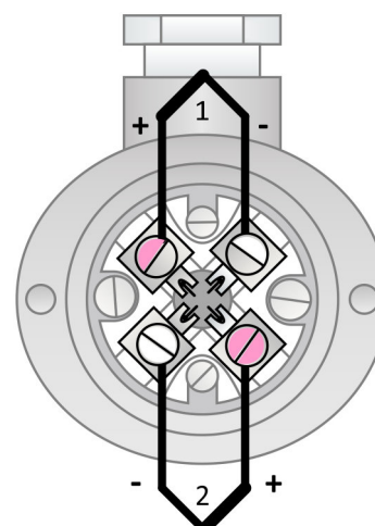
Obrázek 11F.7: Zapojení dvojitého termočláнку
