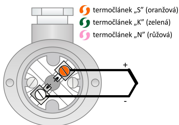
Obrázek 11F.6: Zapojení jednoduchého termočláнку
