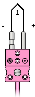
Obrázek 11.9: Zapojení konektoru
