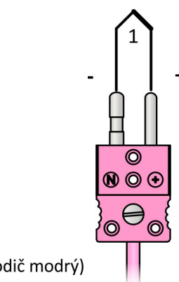
Obrázek 12KP.8: Zapojení konektoru
