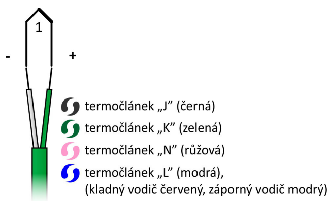
Obrázek 12KP.7: Zapojení jednoduchého termočlátku
