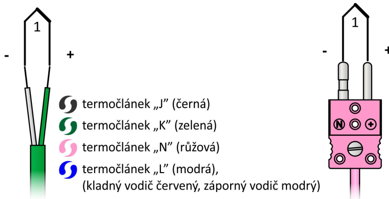
Obrázek 12KR.4: Zapojení jednoduchého termočláunku
