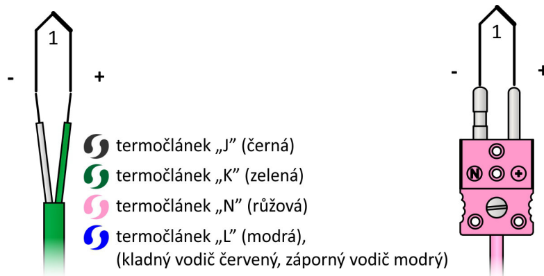
Obrázek 13.3: Zapojení jednoduchého termočláunku
