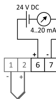
Obrázek 14V.9: zapojení převodníků
