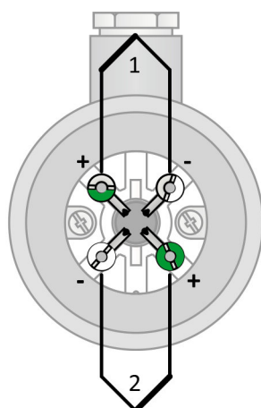
Obrázek 16N.7: zapojení dvojitého termočlánku
