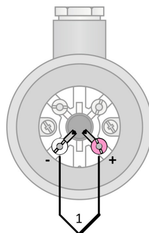
Obrázek 16N.8: zapojení jednoduchého termočlánku
