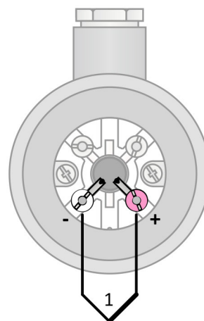
Obrázek 16S.8: zapojení jednoduchého termočlánu
