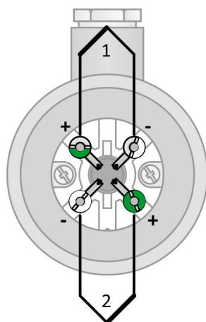
Obrázek 16S.7: zapojení dvojitého termočlánu
