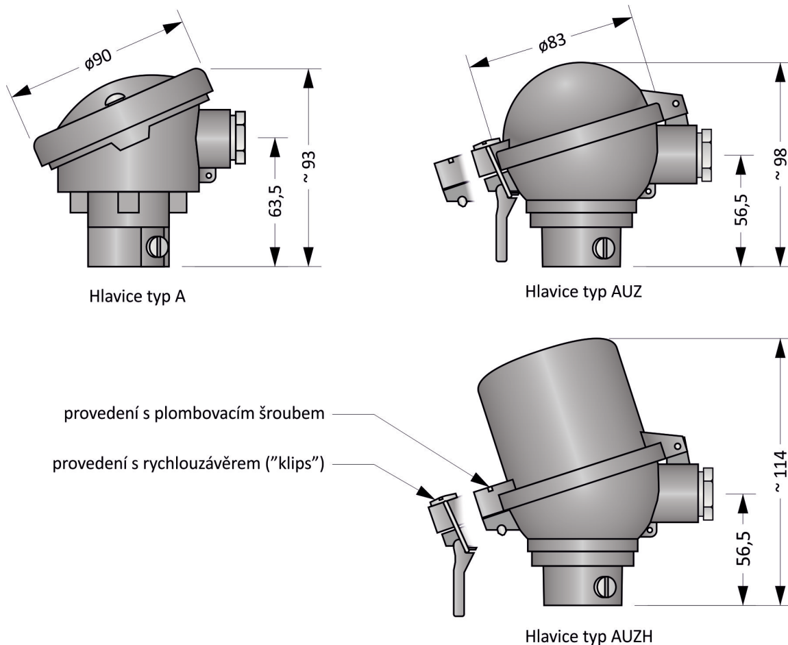
Obrázek 1.2: Typy hlavic
