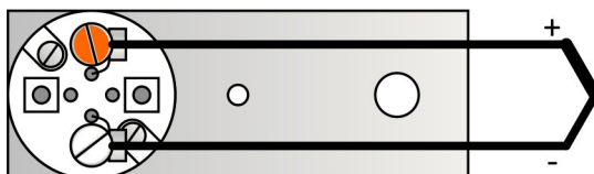
Obrázek 20.2: Schéma zapojení
