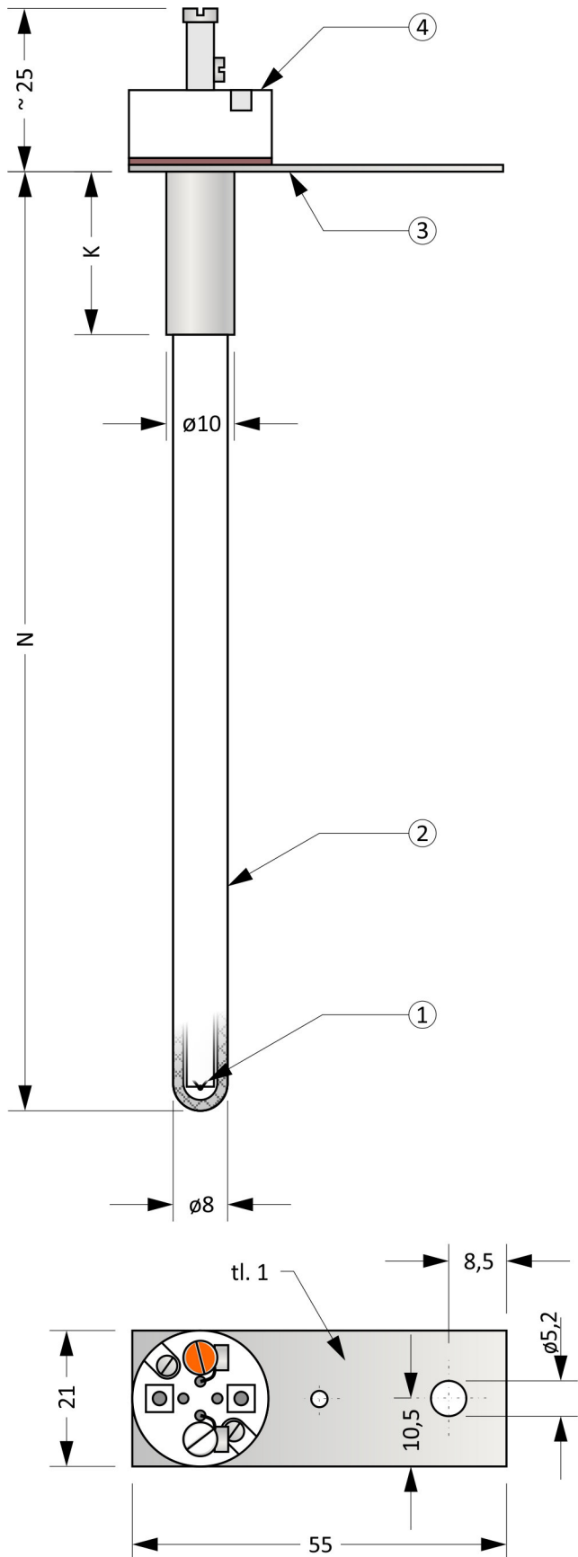
Obrázek 20.1: Snímač MTC20
