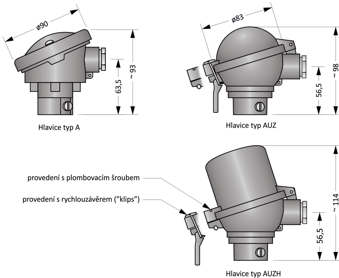
Obrázek 2.2: Typy hlavic
