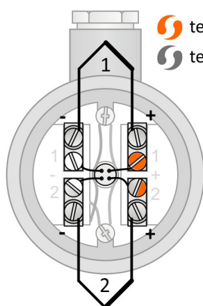
Obrázek 6A.3: zapojení dvojitého termočládku
