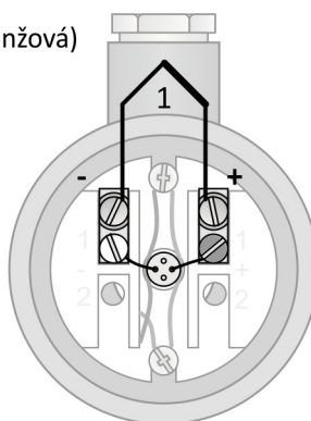
Obrázek 6A.4: zapojení jednoduchého termočládku
