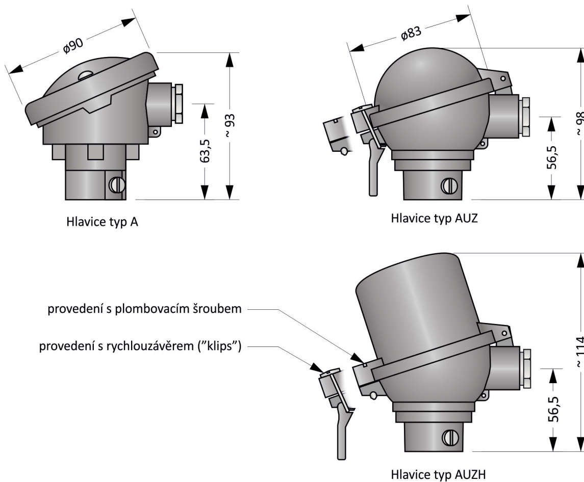
Obrázek 6L.2: Typy hlavic
