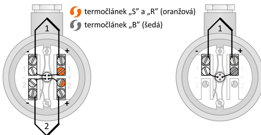
Obrázek 7BM.5: zapojení dvojitého termočláneku
