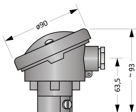
Hlavice typ AB
