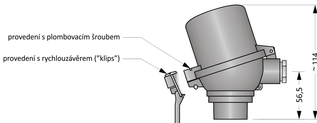
Hlavice typ ABUZH
