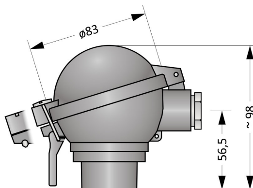
Hlavice typ ABUZ
