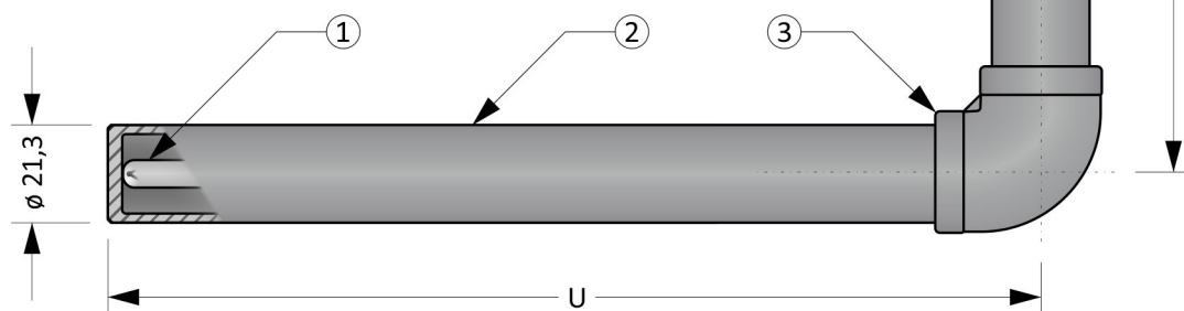
Obrázek 7U.1: MTC7U
