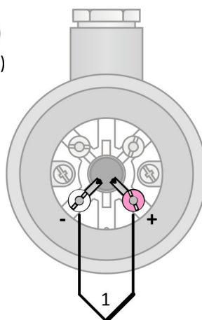
Obrázek 7U.4: zapojení jednoduchého termočlánu
