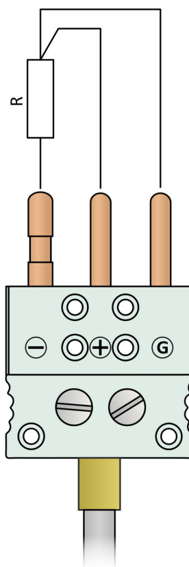
Obrázek 10K.10: RTD v třívodičovém zapojení
