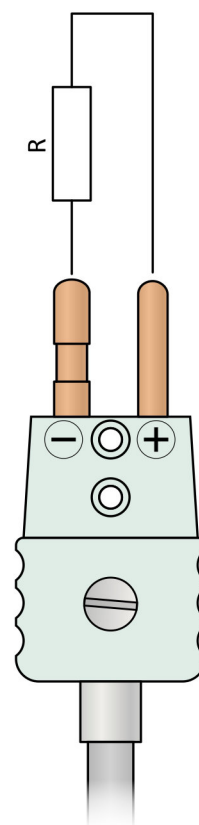
Obrázek 10K.11: RTD v dvou vodičovém zapojení
