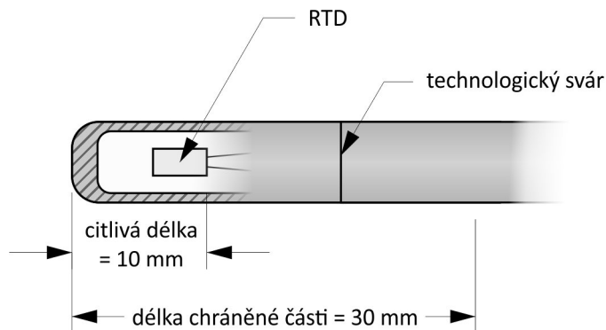
Obrázek 10K.8: detail měřicího konce snímače
