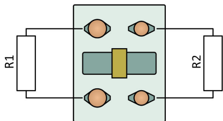
Obrázek 11.15: 2 x RTD v dvou vodičovém zapojení s konektorem
