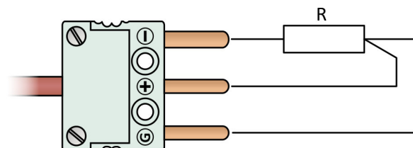
Obrázek 11.20: RTD v třívodičovém zapojení s miniaturním konektorem
