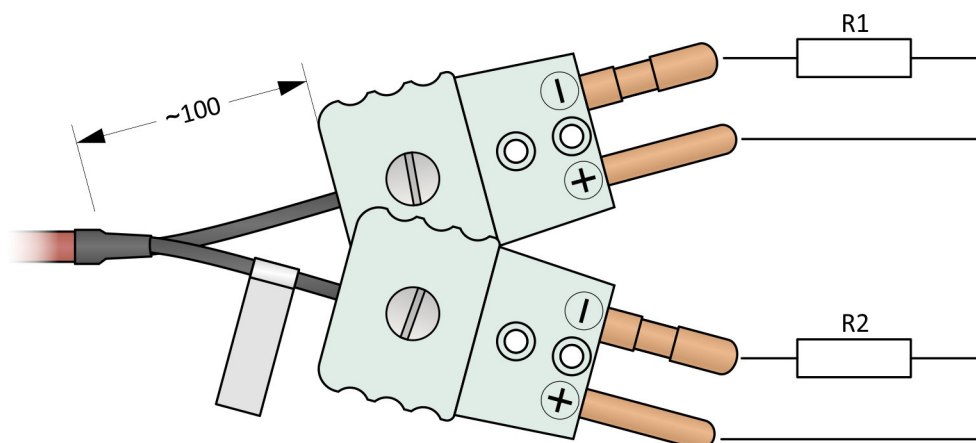
Obrázek 11.21: 2 x RTD v dvouvodičovém zapojení se dvěma konektory
