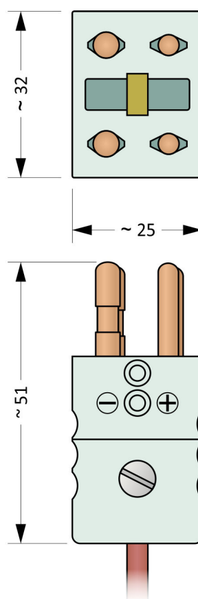
Obrázek 11.7: MTCK-4S
