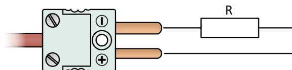
Obrázek 11.19: RTD v dvou vodičovém zapojení s miniaturním konektorem
