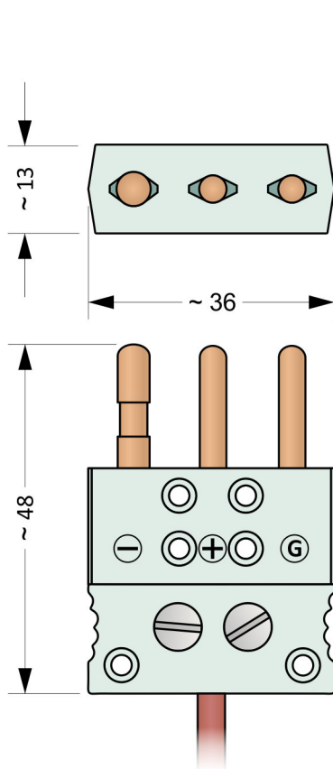
Obrázek 11.6: MTCK-3S
