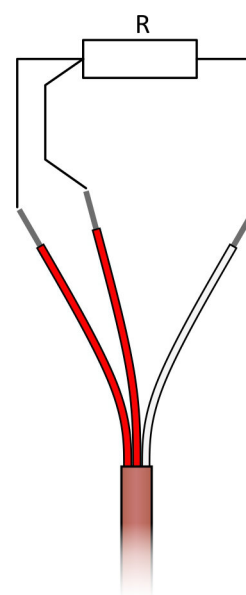
Obrázek 11.9: detail měřicího konce snímače
