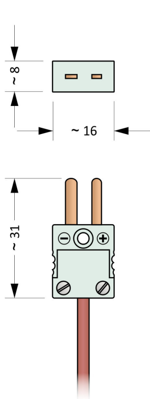
Obrázek 11.3: MTCK-M
