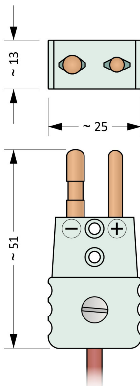
Obrázek 11.4: MTCK-S
