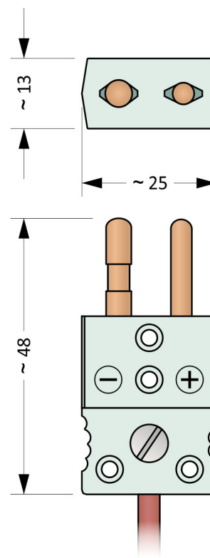
Obrázek 11.5: MTCK-CS
