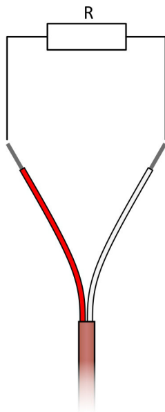
Obrázek 11.11: RTD v dvouvodičovém zapojení
