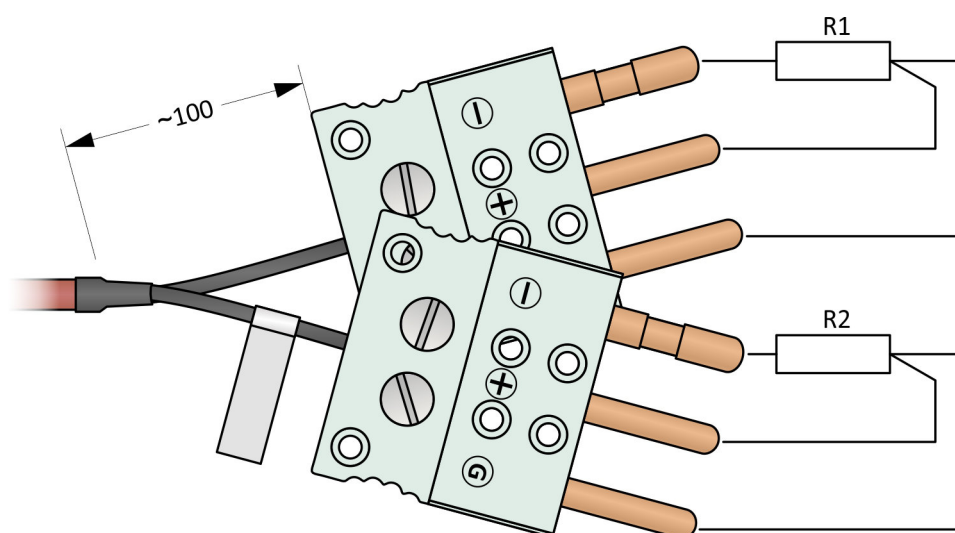
Obrázek 11.22: 2 x RTD v třívodičovém zapojení se dvěma konektory
