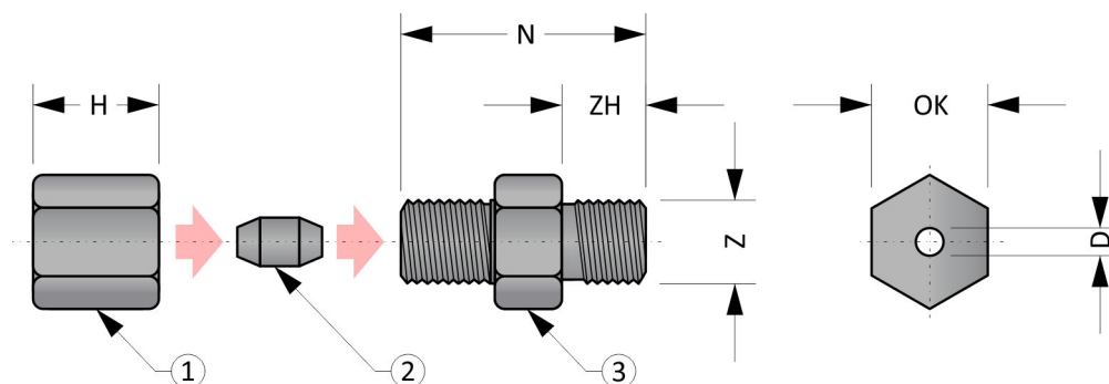
Obrázek PS.2: Posuvné šroubení s oválnou kleštinou
