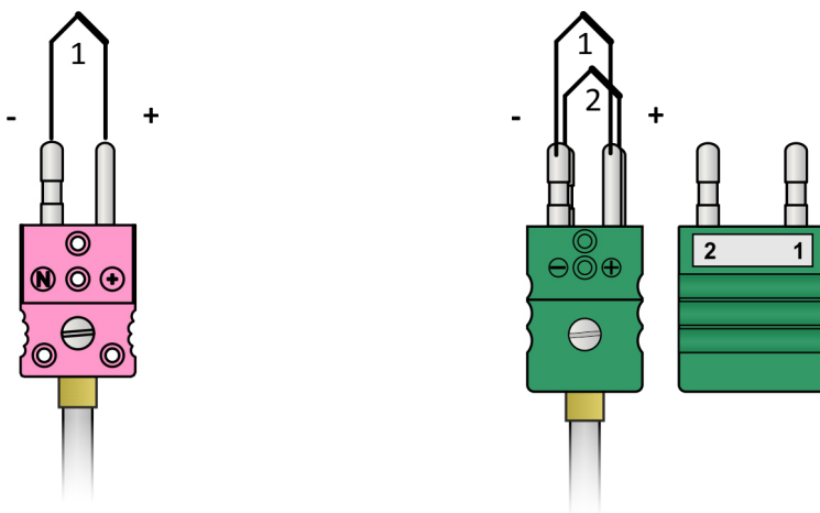
Obrázek 10.8: Zapojení konektoru
