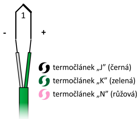
Obrázek 11R.7: Zapojení jednoduchého termočláňku
