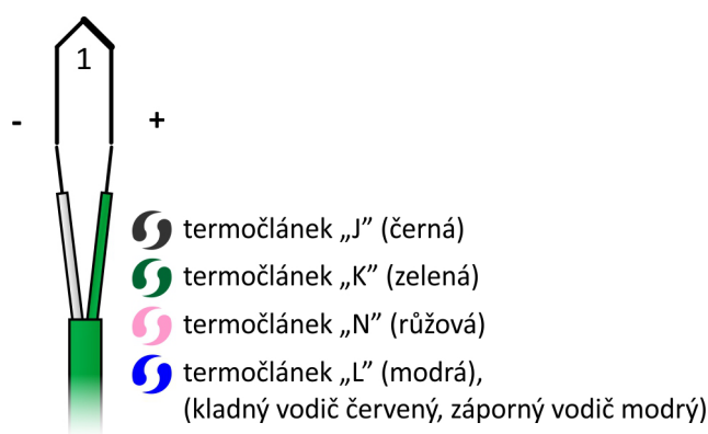
Obrázek 12KP.7: Zapojení jednoduchého termočlánu
