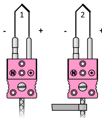
Obrázek 1KV.6: zapojení konektoru
