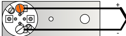
Obrázek 20.2: Schéma zapojení
