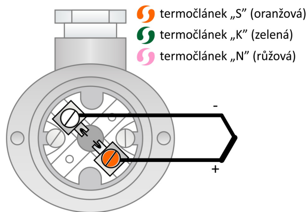
Obrázek 22.2: Schéma zapojení
