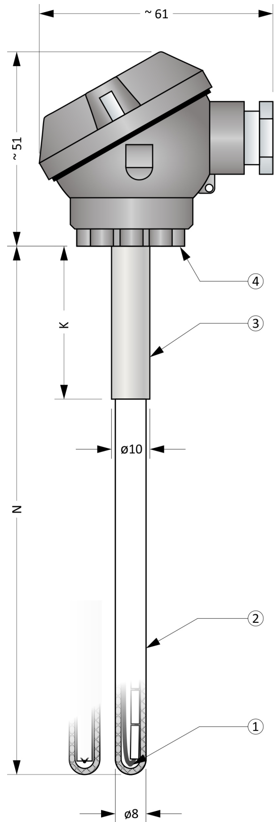
Obrázek 22.1: Snímač MTC22
