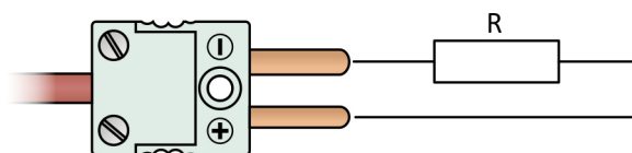
Obrázek 11.17: RTD v dvou vodičovém zapojení s miniaturním konektorem
