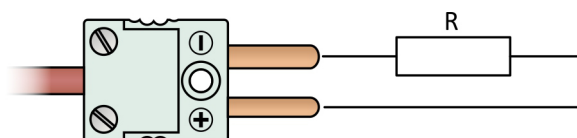
Obrázek 12.17: RTD v dvou vodičovém zapojení s miniaturním konektorem
