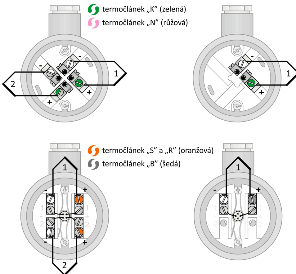
Obrázek 1KD.3: zapojení dvojitého termočlásku
