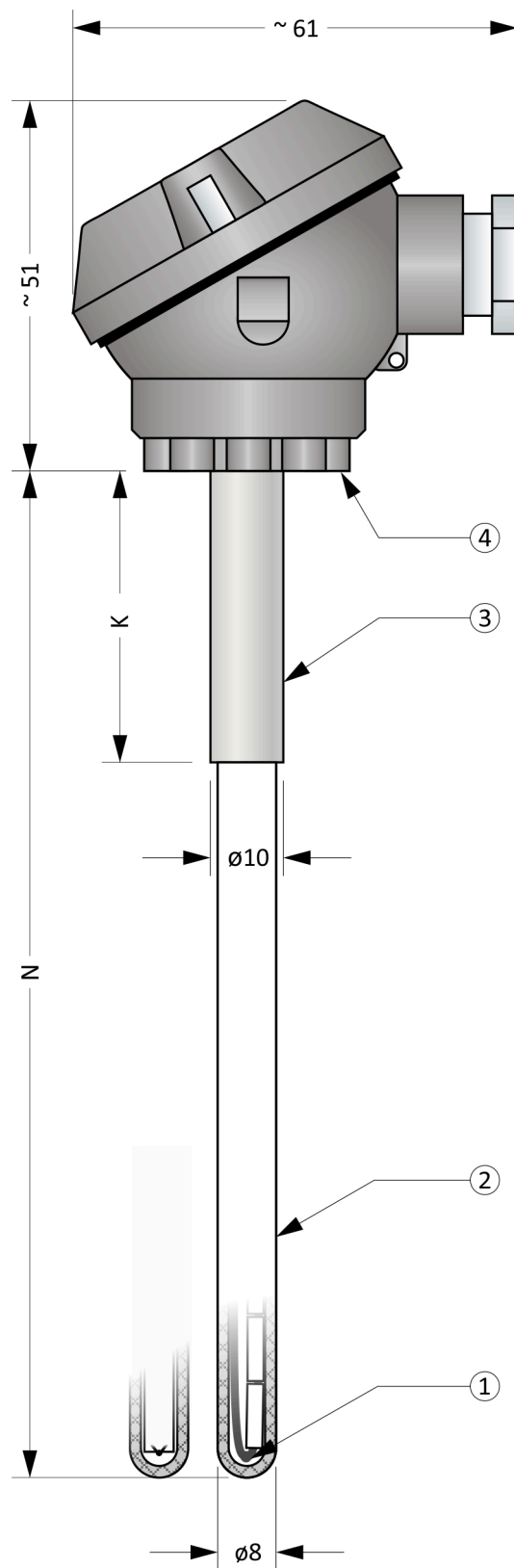
Obrázek 22.1: Snímač MTC22
