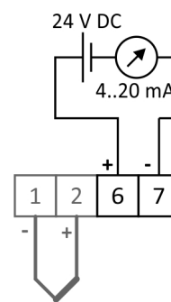
Obrázek 9.5: zapojení převodníků
