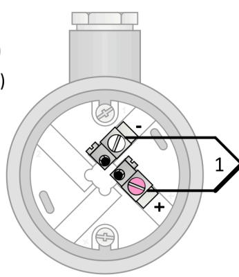
Obrázek 9.4: zapojení jednoduchého termočlánu
