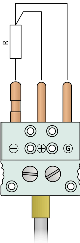
Obrázek 10K.10: RTD v třívodičovém zapojení
