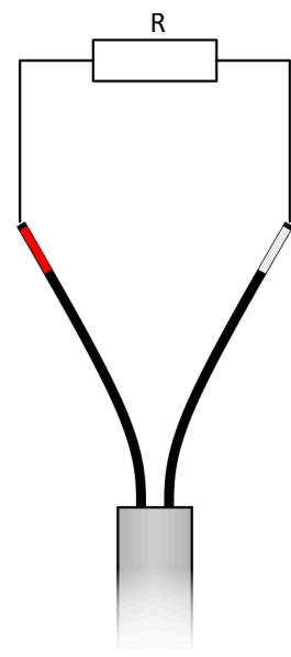
Obrázek 10.5: RTD v dvouvodičovém zapojení
