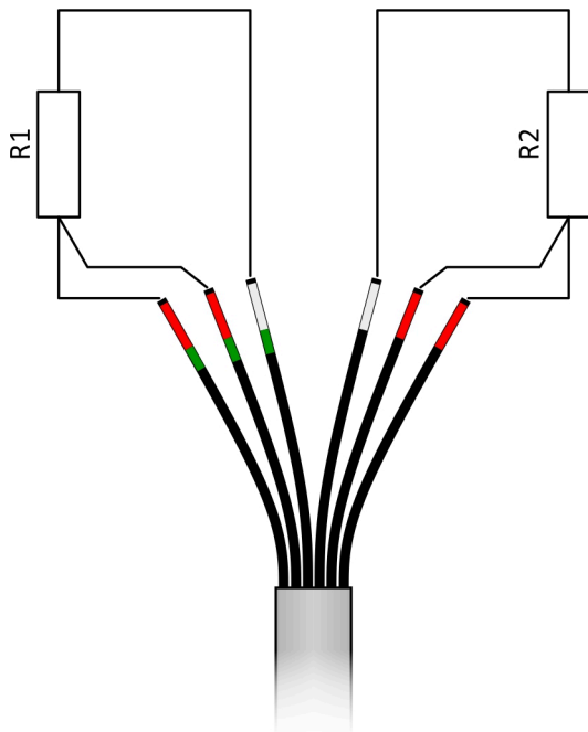
Obrázek 10.6: 2 x RTD v třívodičovém zapojení
