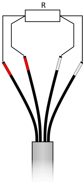
Obrázek 10.3: RTD v čtyřvodičovém zapojení
