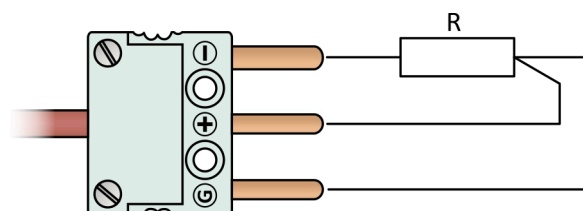
Obrázek 11.20: RTD v třívodičovém zapojení s miniaturním konektorem
