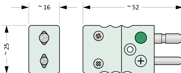
Obrázek MK.CS.1: konektor MTCK-CSM-K
