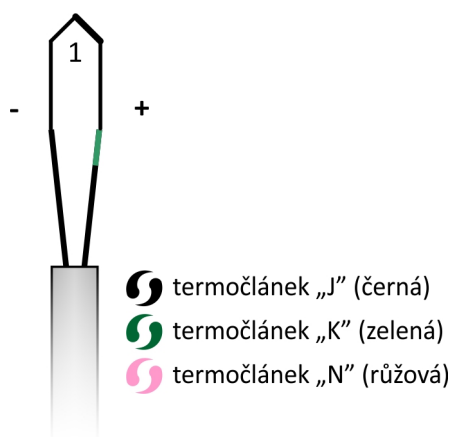
Obrázek 10.6: Zapojení jednoduchého termočláňku
