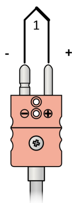
Obrázek 10.8: Zapojení konektoru
