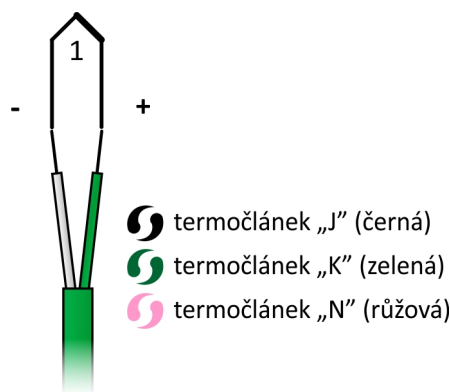
Obrázek 11R.7: Zapojení jednoduchého termočláнку
