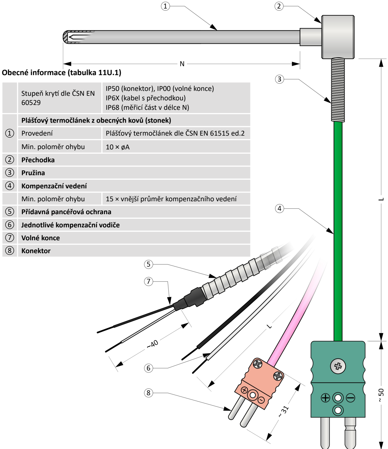
Obrázek 11U.1: MTC11U
