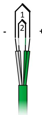
Obrázek 11U.8: Zapojení dvojitého termočláneku
