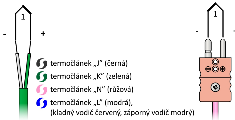
Obrázek 12A.2: Zapojení jednoduchého termočlánku
