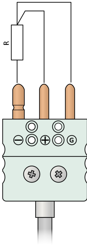
Obrázek 10K.10: RTD v třívodičovém zapojení u standardního konektoru
