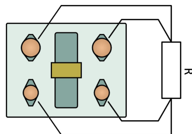
Obrázek 10K.14: RTD v čtyřvodičovém zapojení u standardního konektoru
