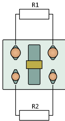
Obrázek 10K.13: 2 x RTD v dvou vodičovém zapojení u standardního konektoru
