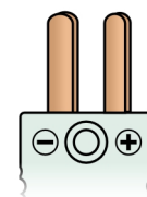
Obrázek 10K.16: RTD v čtyřvodičovém zapojení u miniaturního konektoru
