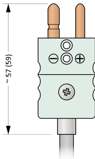
Obrázek 10K.2: MTCK-S (MTCK-CS)
