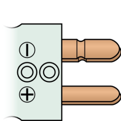
Obrázek 10K.13: 2 x RTD v dvou vodičovém zapojení u standardního konektoru
