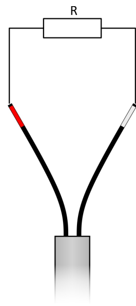
Obrázek 10.5: RTD v dvouodičovém zapojení
