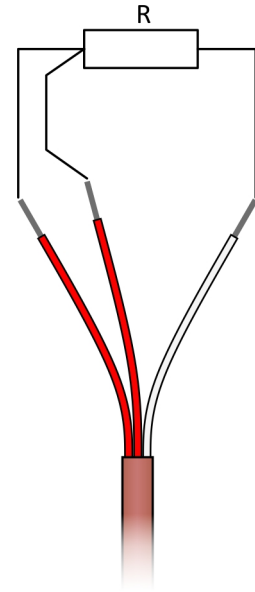
Obrázek 11R.13: RTD v třívodičovém zapojení
