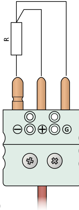
Obrázek 11R.15: RTD v dvou vodičovém zapojení s miniaturním konektorem
