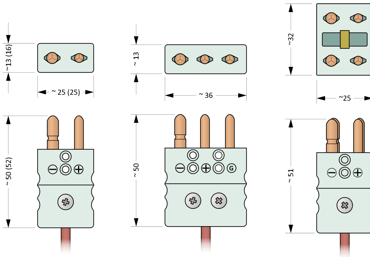
Obrázek 11R.4: MTCK-S (MTCK-CS)
