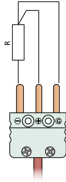
Obrázek 11.16: RTD v třívodičovém zapojení s miniaturním konektorem
