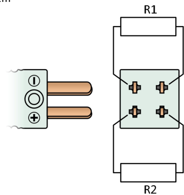
Obrázek 11.19: 2 x RTD v dvou vodičovém zapojení s miniaturním konektorem
