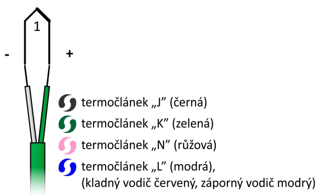
Obrázek 13T.2: Zapojení jednoduchého termočlánu
