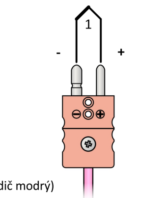
Obrázek 13.4: Zapojení konektoru
