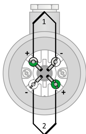
Obrázek 15.4: zapojení dvojitého termočláňku
