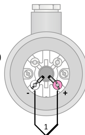
Obrázek 15.5: zapojení jednoduchého termočláňku
